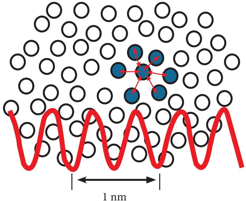
Bir molekülün titreşimi iletimi ve dalga boyu şekillenmesi
