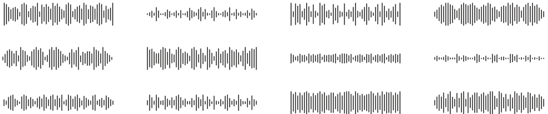
Çeşitli seslere ait titreşimlerin frekans desenleri
